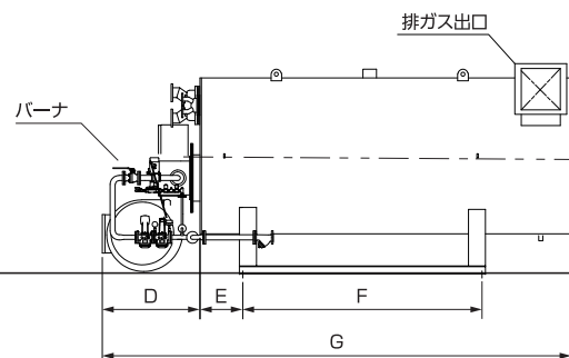
側面図
