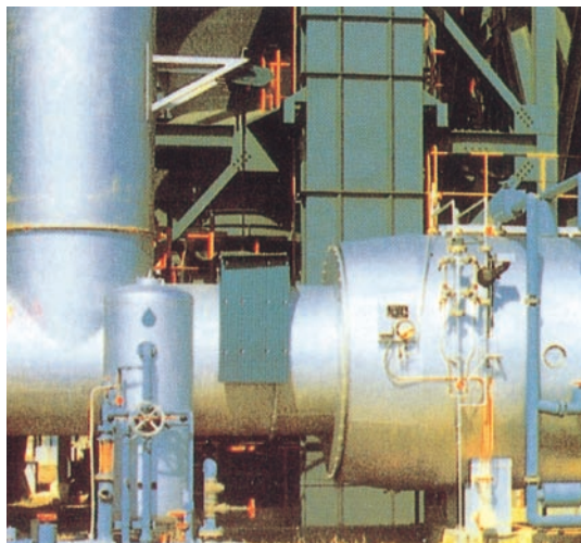
横置型煙管式廃熱ボイラ
